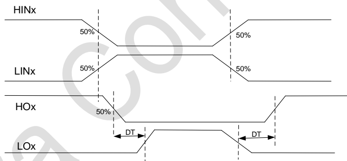
图 5-10 死区功能
