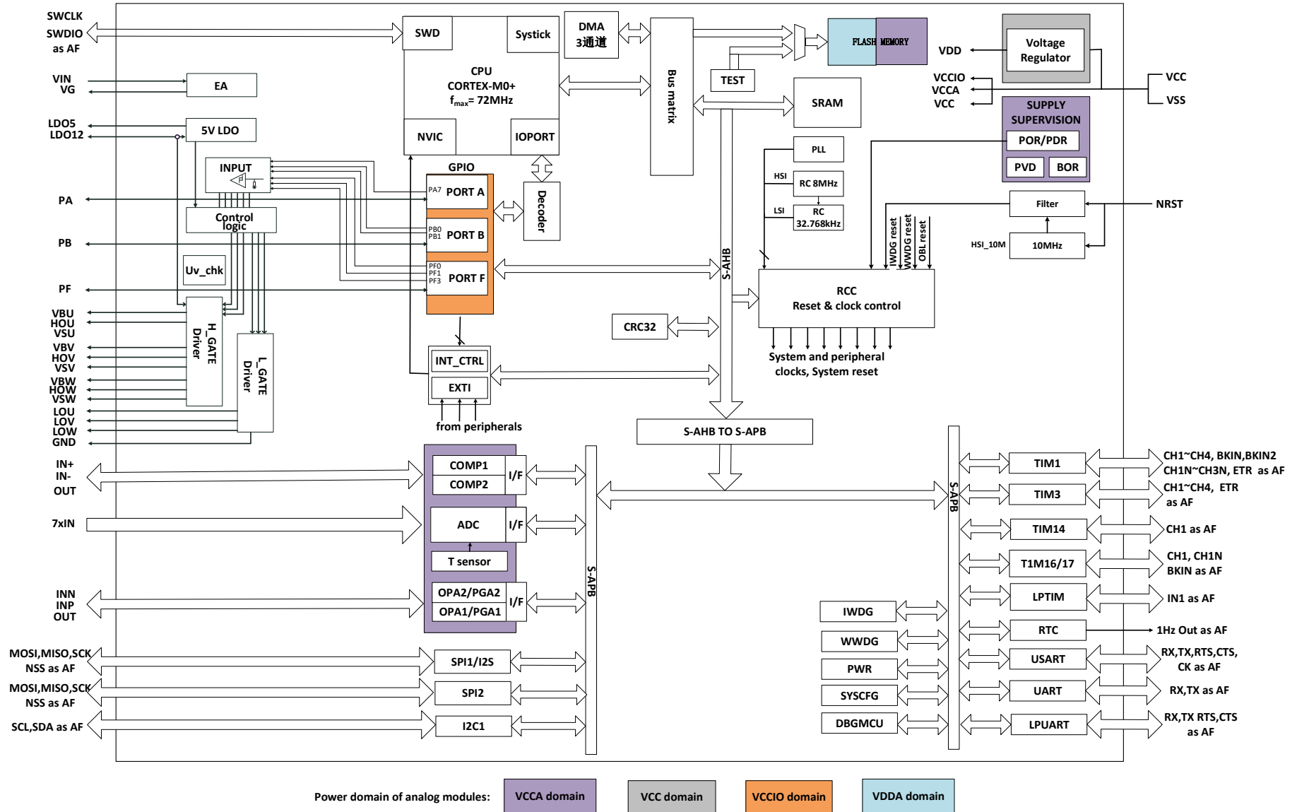
图 1-1 功能模块
