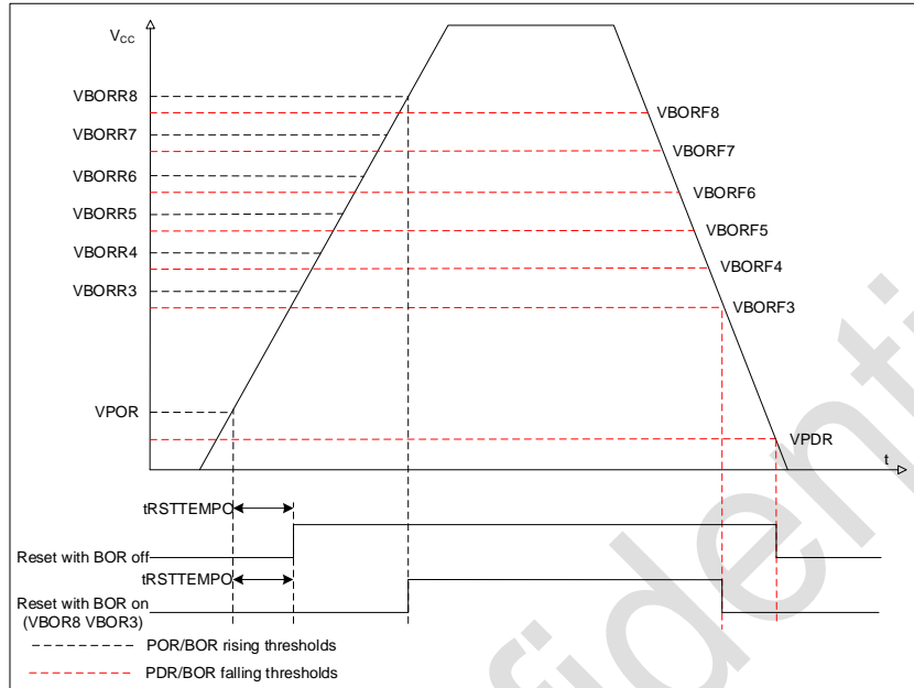
图 2-4 POR/PDR/BOR 阈值
