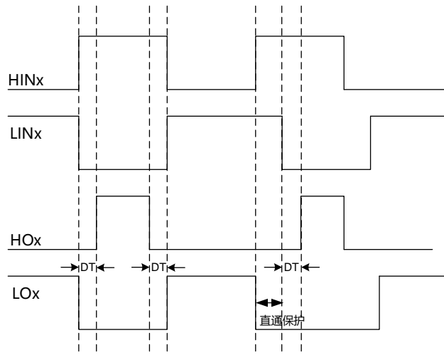
图 5-9 直通保护
